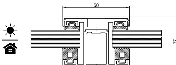
PROFIL ŚRODKOWY PIONOWY
