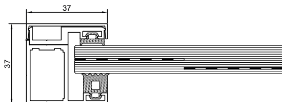
PROFIL BOCZNY PIONOWY
