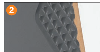
2 Nakładka zewnętrzna z wodoodpornego materiału HDF o grubości 12 mm. Hybrydowe połączenie nakładki zewnętrznej z ramą skrzydła PVC tworzy jednolitą powierzchnię skrzydła o głębokości 94 mm.
