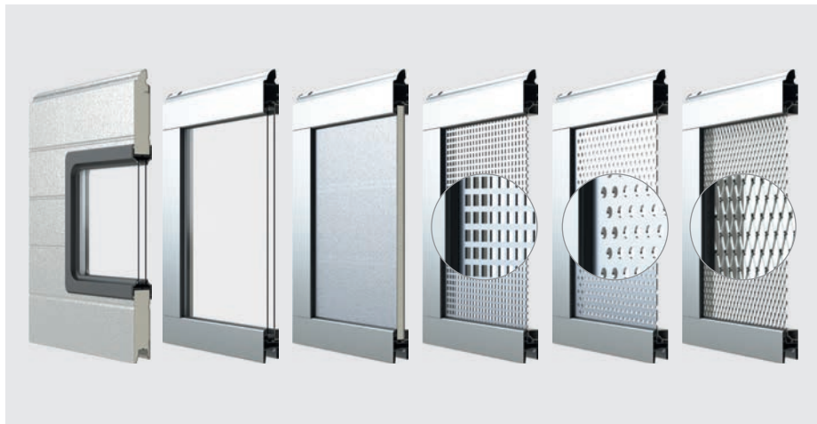
SEKCJE SPECJALNE (od lewej): IS/A z oknami, IP z podwójną szybą, IP z przekładką, IP z blachą perforowaną, IP z siatką alu.
